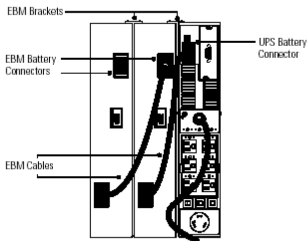
Рисунок 27. Подключение ВБМ
