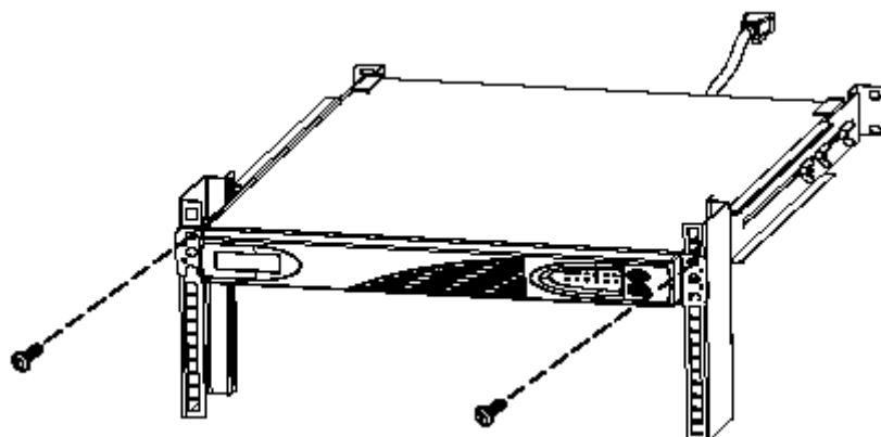
Рисунок 6. Закрепление ИБП в 19 “ стойке
