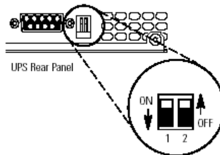
Рисунок 14. DIP переключатели
