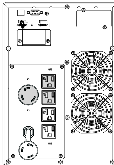
Рисунок 46. Модель PW9130L2000T-XL
