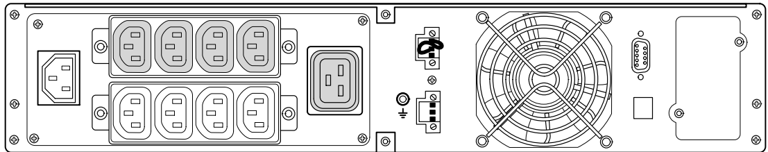
Рисунок 37. Модели PW9130i2000R-XL2U, PW9130G2000R-XL2UEU
