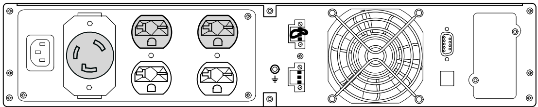
Рисунок 36. Модель PW9130G2000R-XL2U
