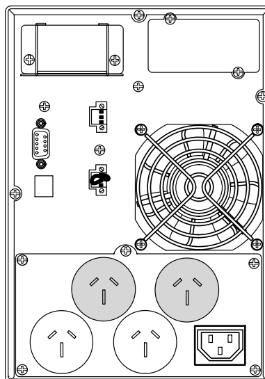
Рисунок 58. Модель PW9130G1500T-XLAU
