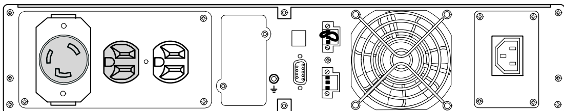
Рисунок 29. Модель PW9130G1000R-XL2U
