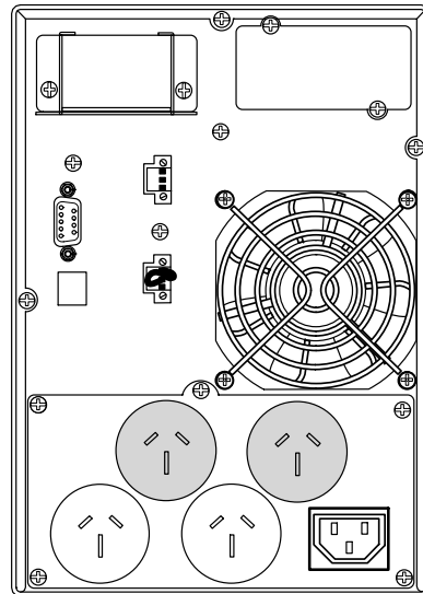
Рисунок 58. Модель PW9130G1500T-XLAU
