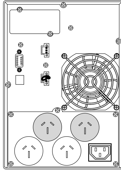
Рисунок 56. Модель PW9130G700T-XLAU
