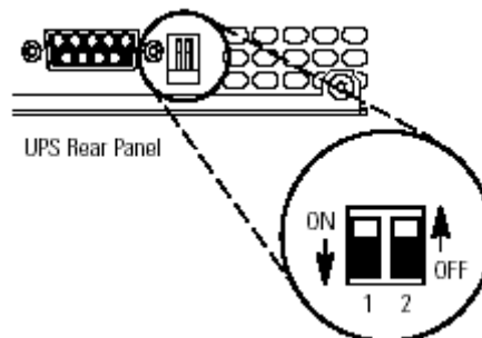
Рисунок 14. DIP переключатели
