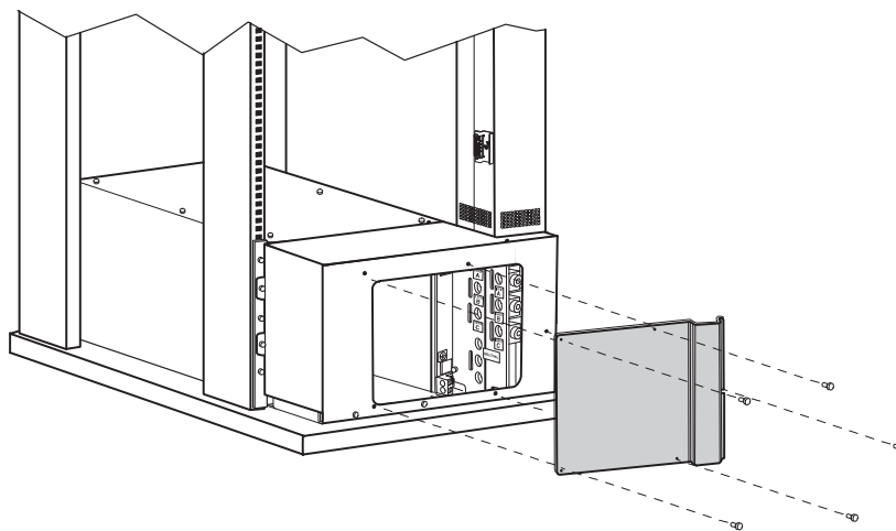
Рисунок 5. Снятие крышки кабельного канала (стойка с нижним вводом)
