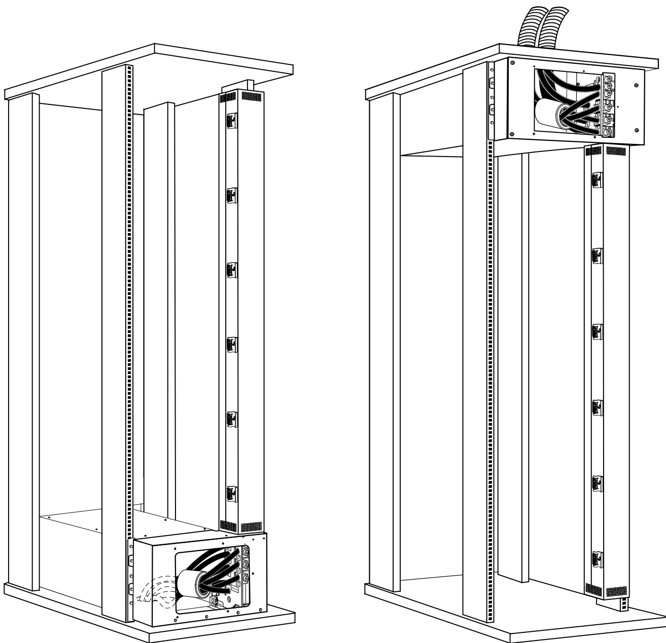
Проводка в стойке с верхним вводом
