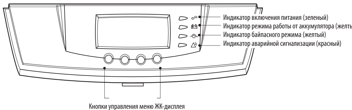
Рисунок 45. Панель управления модуля BladeUPS
