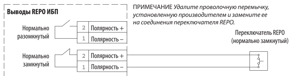
Рисунок 53. Подключение нормально замкнутого REPO в автономном ИБП
