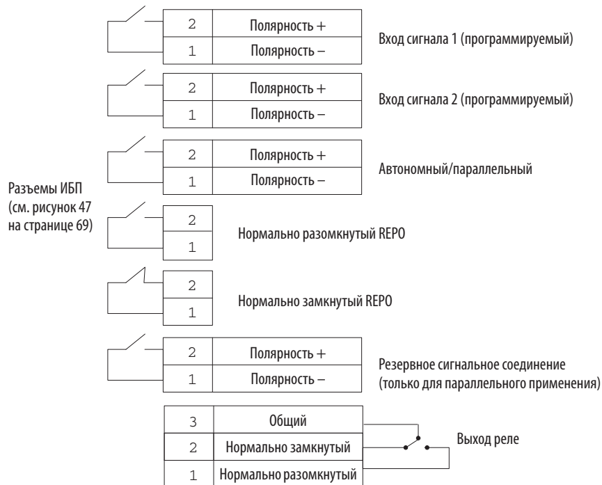
Рисунок 51. Внешние подключения управляющих выводов
