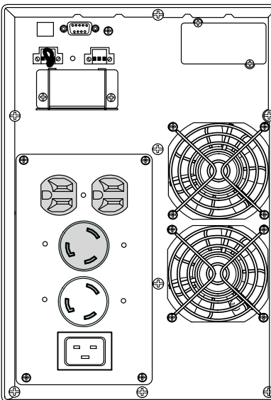
Рисунок 50. Модель PW9130G3000T-XL
