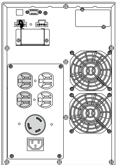
Рисунок 49. Модель PW9130G2000T-XL
