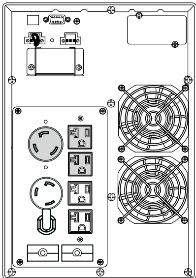
Рисунок 47. Модель PW9130L3000T-XL
